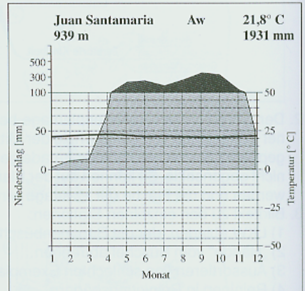
M 4: Klimadiagramm von Juan Santamaria in Costa Rica
